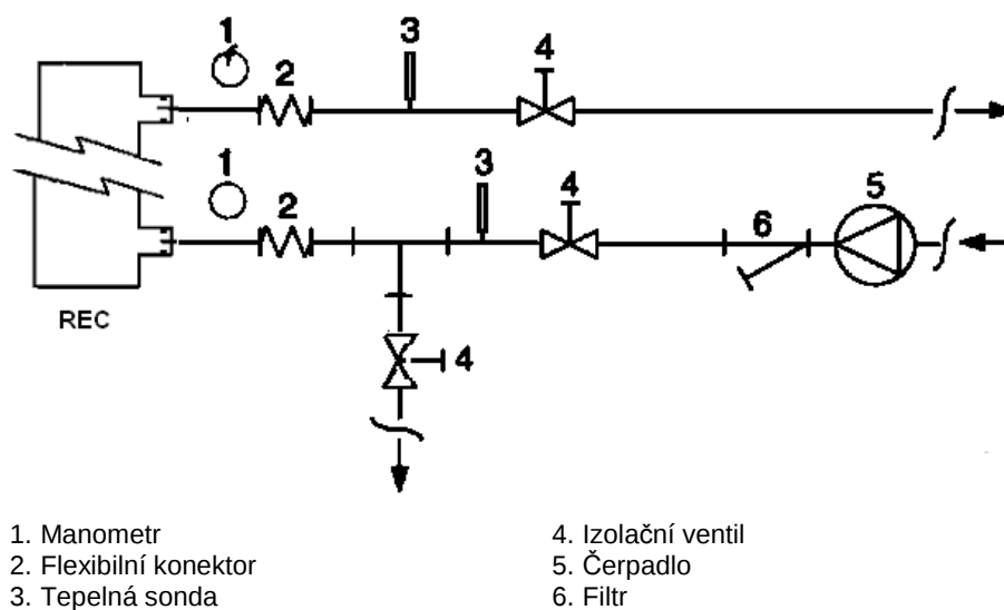
Obrázek 6 - Zapojení vodních trubek k výměníkům rekuperace tepla
