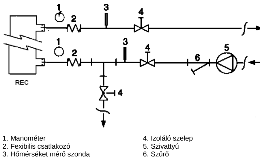
Ábra 6 - Vízvezetékek bekötése a hővisszanyerő hőcserélőkhöz
