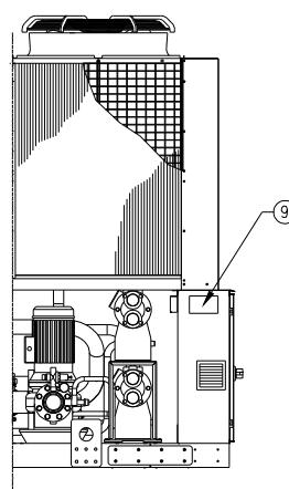
Εικόνα 1 – Περιγραφή των ετικετών που εφαρμόζονται στον ηλεκτρικό πίνακα
