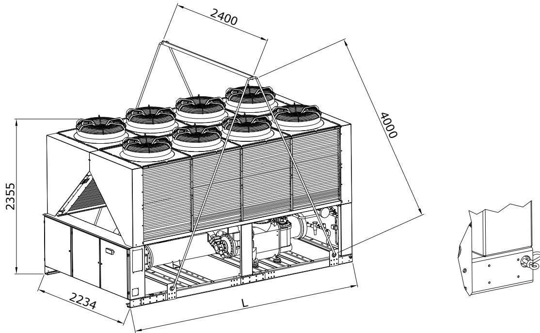
Kuva 3 – Yksikön nostaminen
