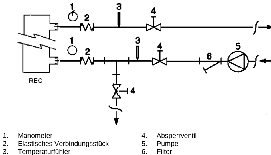
Abbildung 6 - Anschluss der Wasserleitungen an die Rückgewinnungswärmetauscher
