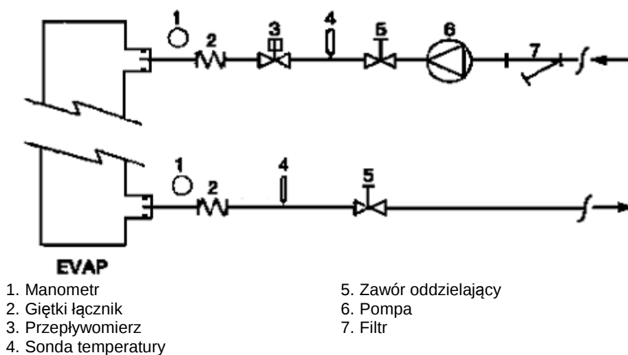
Rysunek 6 - Podłączenie rur wodnych do wymienników ciepła
