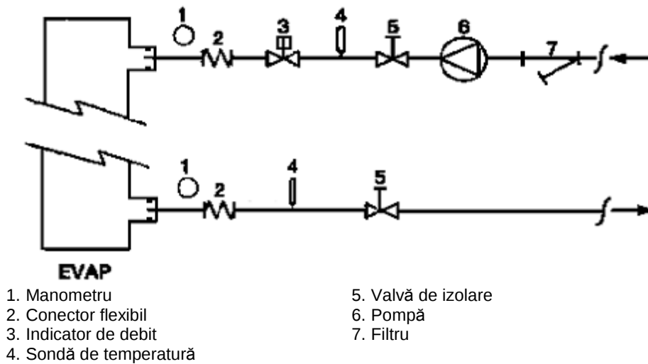
Figura 6 - Conectarea tuburilor de apă pentru schimbătoarele de recuperare a căldurii
