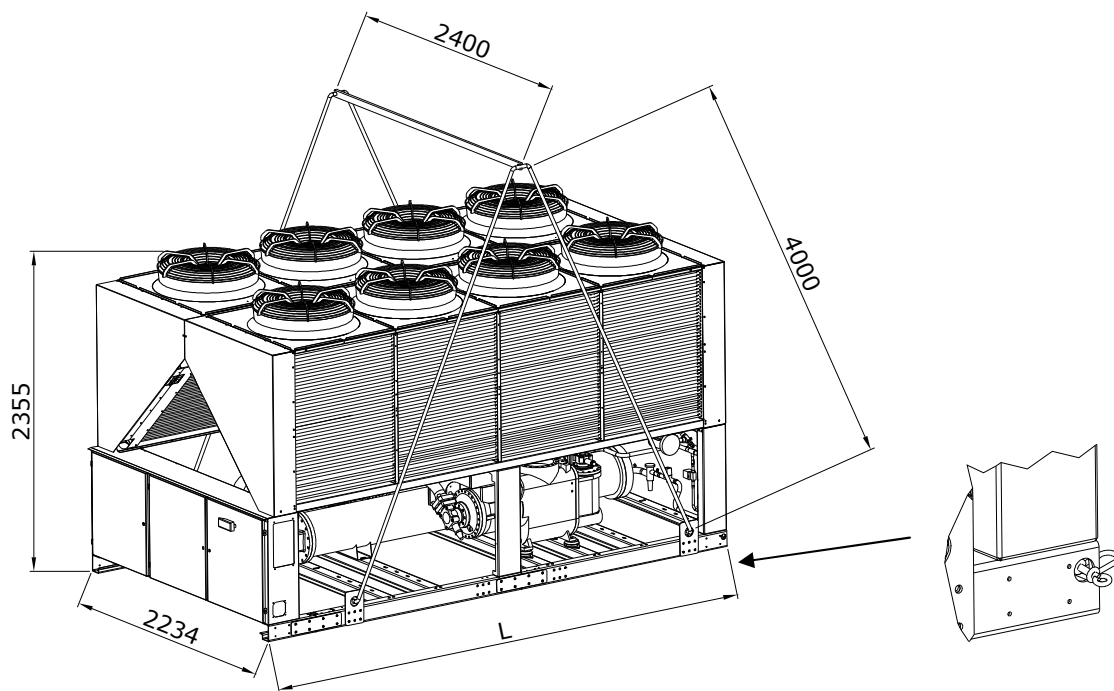
Figura 3 – Sollevamento dell'unità
