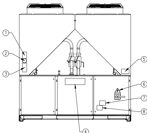
Ábra 1 – Az elektromos burokaltoakra elhelyezett címkék értelmezése
