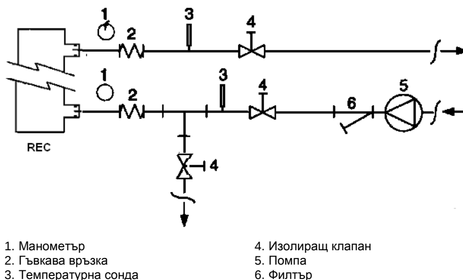
Схема 6 – Свързване на тръбите за вода за топлообменниците за топлинна енергия
