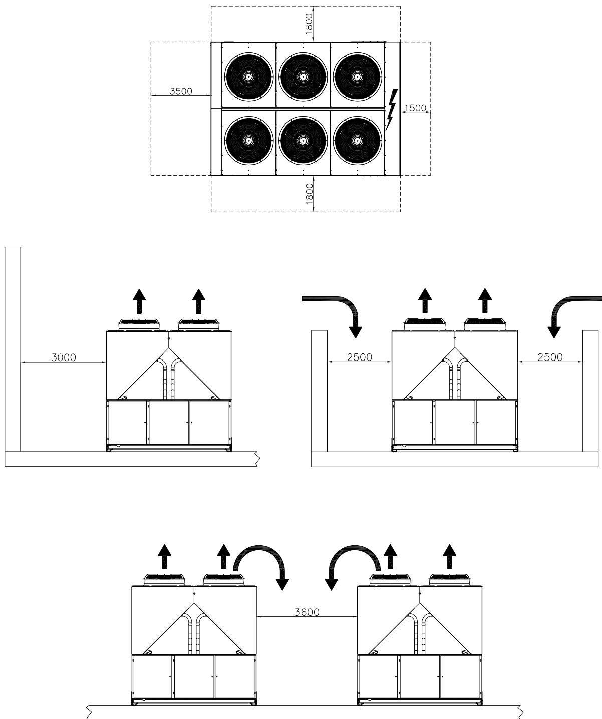
Figura 4 – Requisiti di spazio minimi
