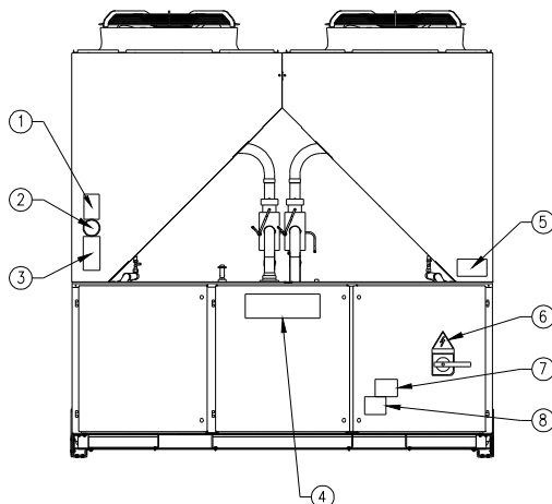
Figuur 1 – Beschrijving van de etiketten op het elektrische paneel
