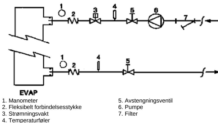
Figur 6 – Forbindelse av vannledninger for vekslerer for varmegjenvinning
