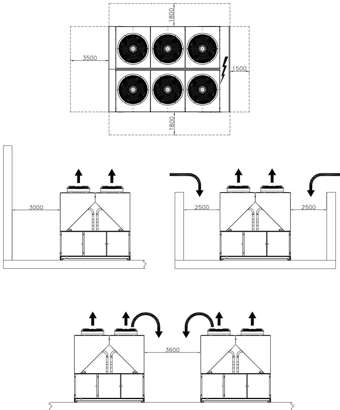
Abbildung 4 – Mindestabstände
