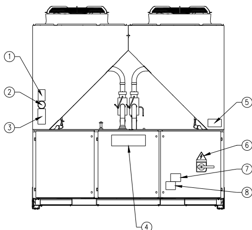
Figura 1 – Descrierea etichetelor aplicate pe tabloul electric
