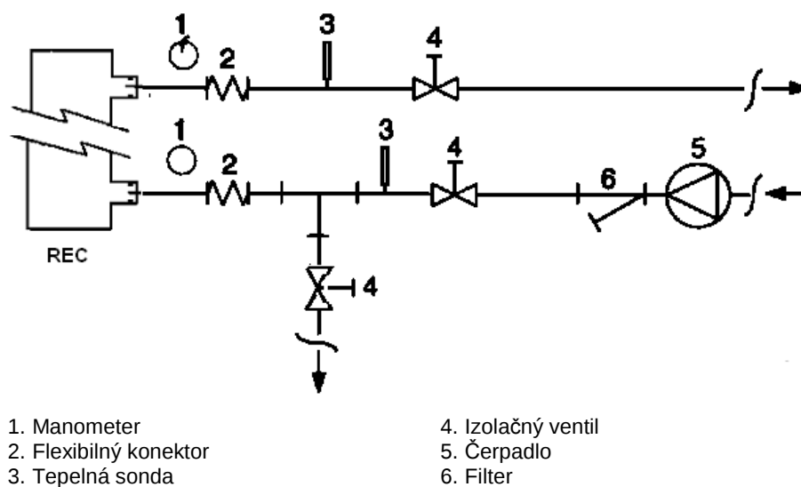
Obrázok 6 - Zapojenie vodných trubiek k výmenníkom rekuperácie tepla
