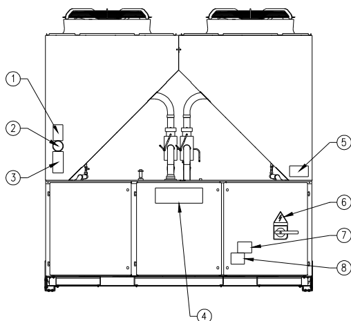
Slika 1 – Opis nalepk na električni omarici
