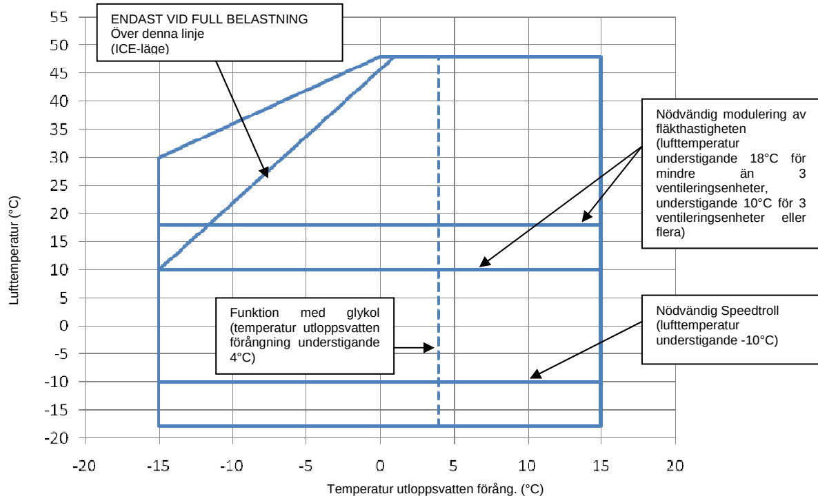
Figur 2 – Operativa begränsningar
