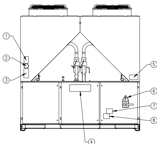
Figure 1 – Description des étiquettes appliquées sur le tableau électrique
