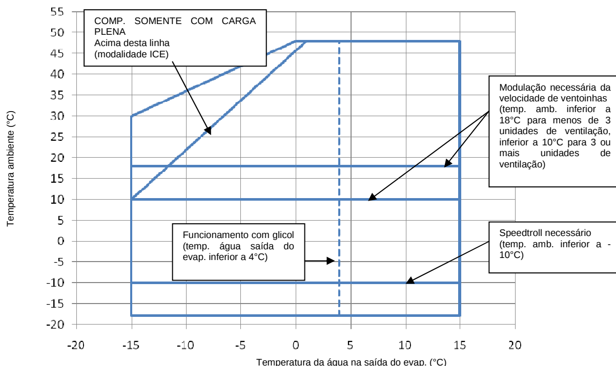
Figura 2 – Limites operativos
