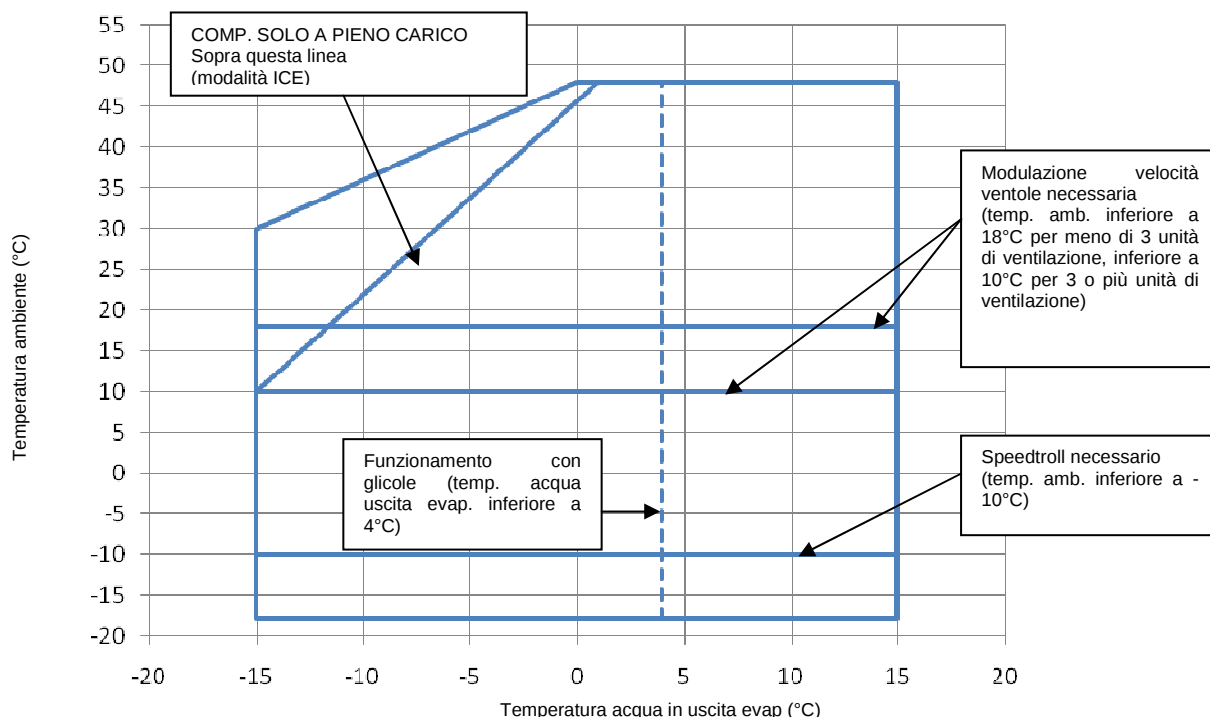
Figura 2 – Limiti operativi
