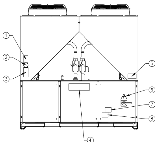
Рисунок 1 – Описание табличек, установленных на электрической панели агрегата
