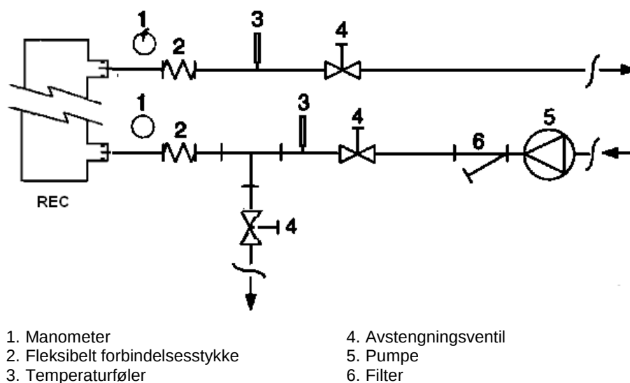
Figur 6 – Forbindelse av vannledninger for vekslerer for varmegjenvinning
