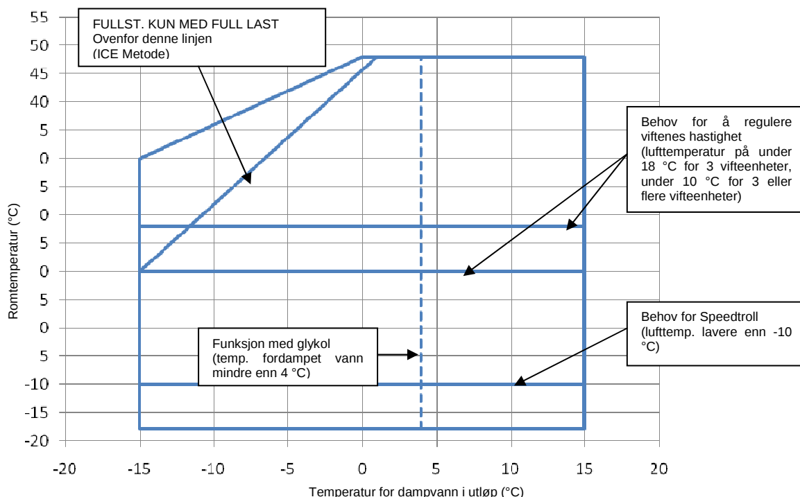
Figur 2 - Belastningskapasitet
