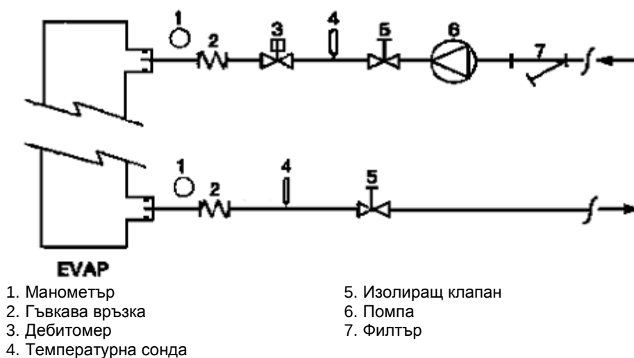
Схема 6 – Свързване на тръбите за вода за топлообменниците за топлинна енергия
