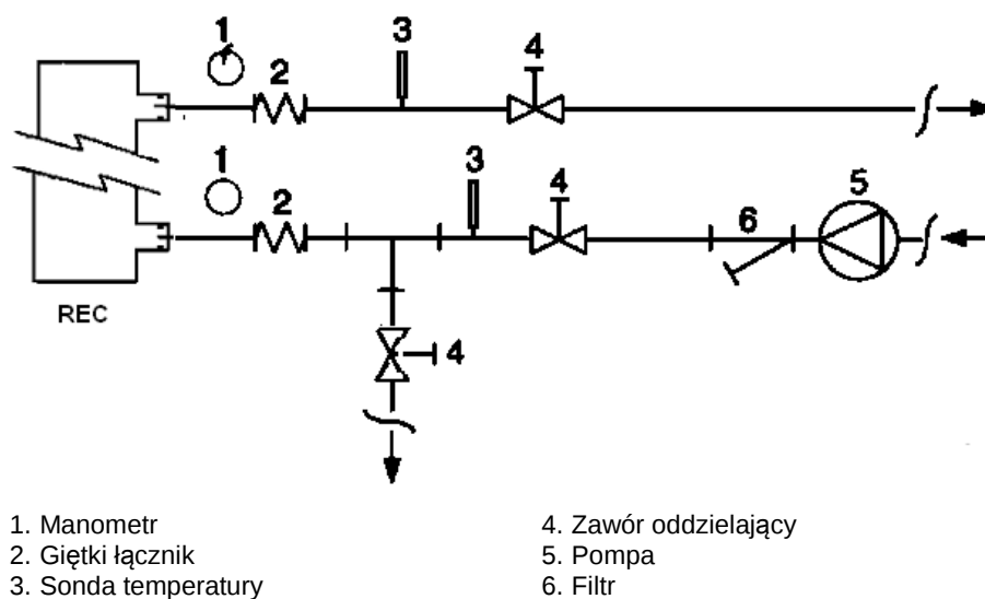
Rysunek 6 - Podłączenie rur wodnych do wymienników ciepła
