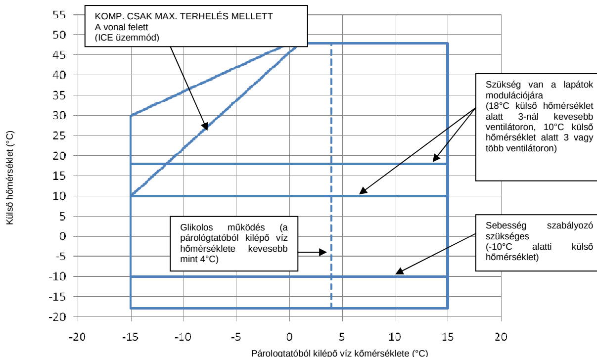
Ábra 2 – Üzemi tartomány
