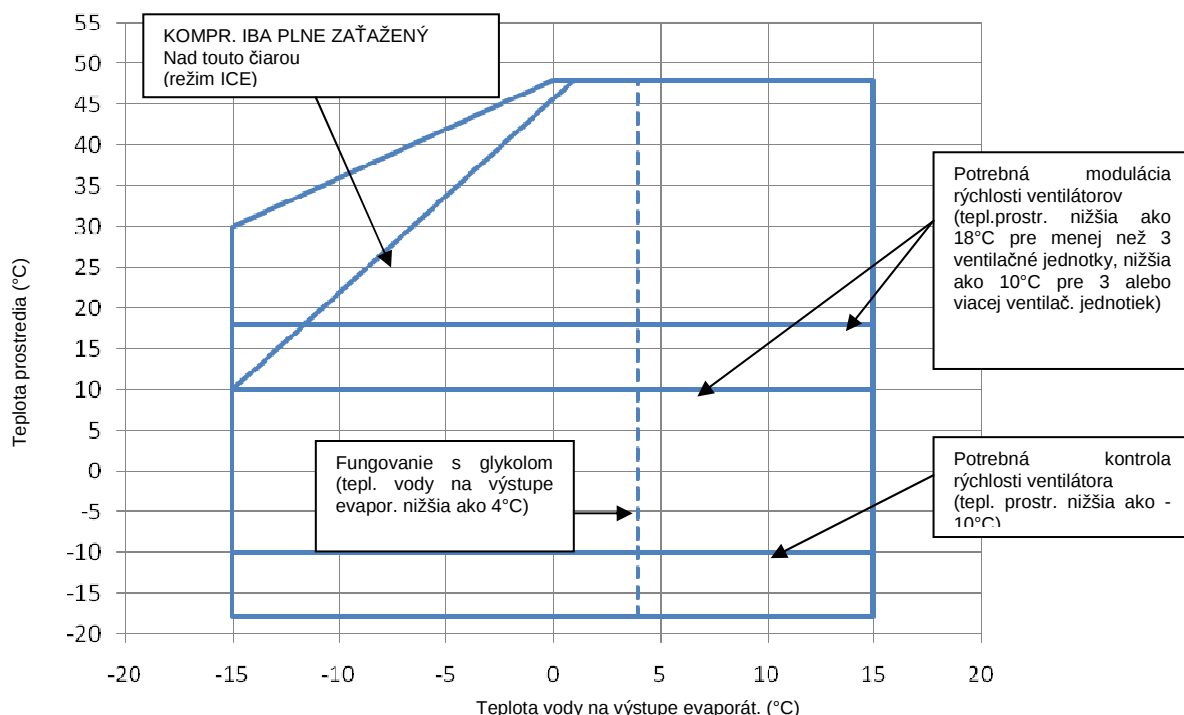
Obrázok 2 - Operačné limity
