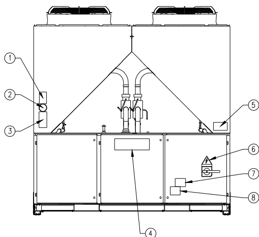
Figura 1 – Descrizione delle etichette applicate al pannello elettrico
