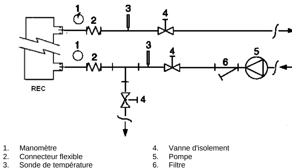
Figure 6 - Raccordement des tuyaux d'eau pour les échangeurs de récupération de chaleur
