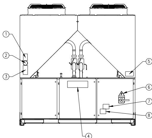
Abbildung 1 – Am Schaltschrank angebrachte Klebeschilder
