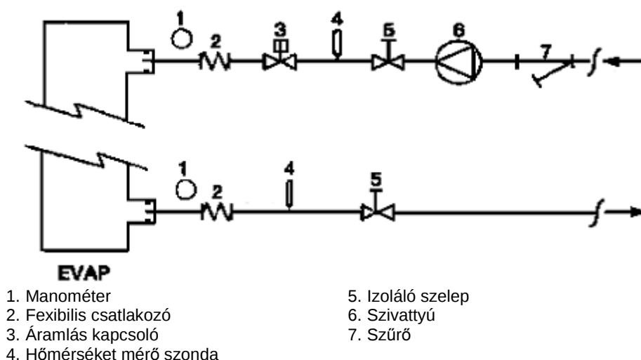
Ábra 6 - Vízvezetékek bekötése a hővisszanyerő hőcserélőkhöz
