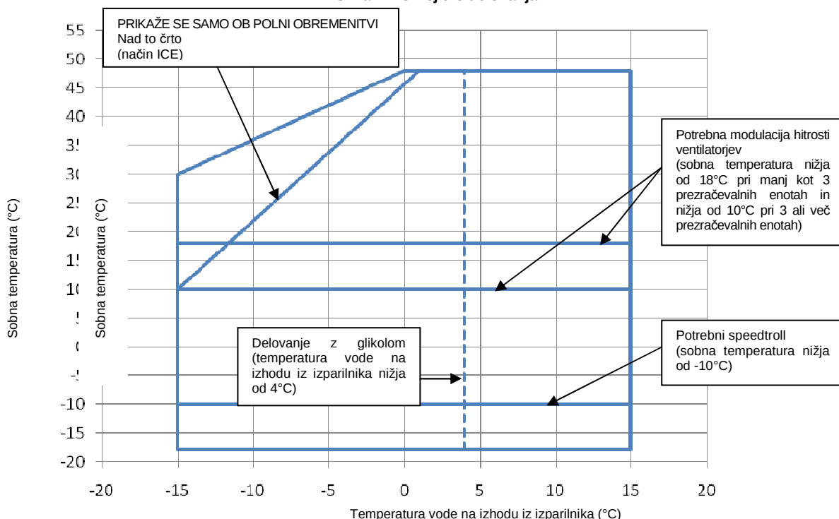
Slika 2 – Omejitve delovanja
