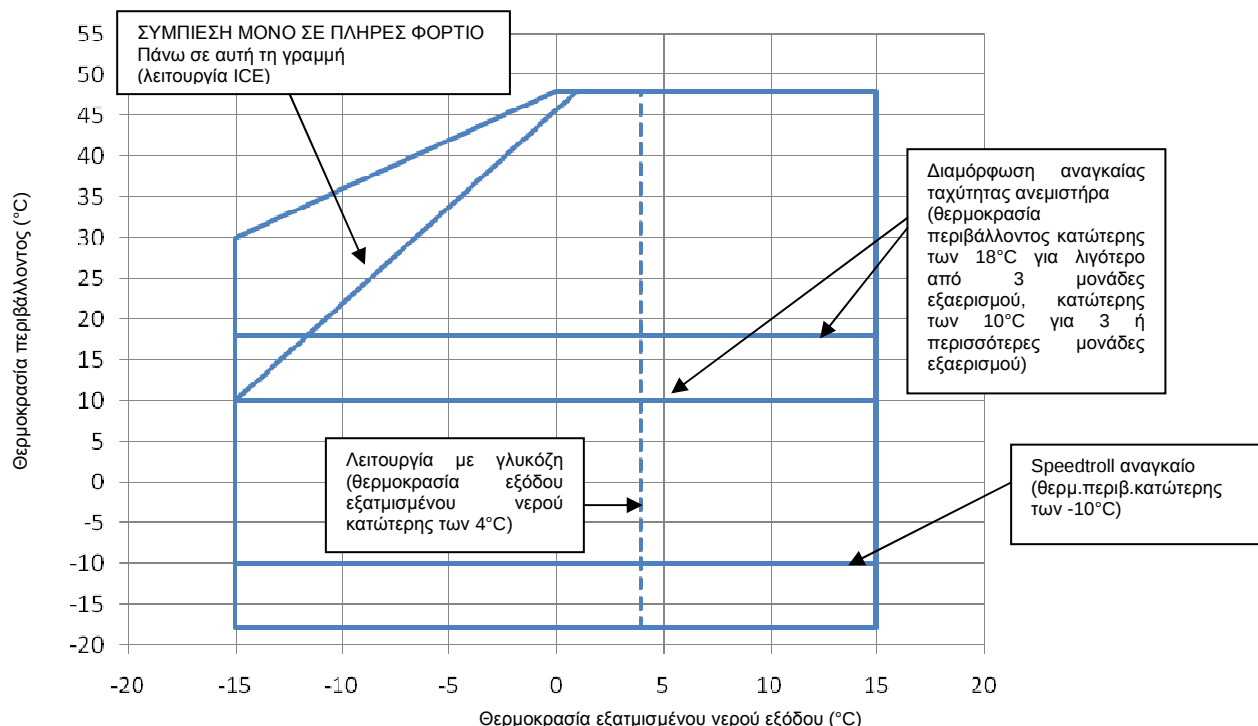
Εικόνα 2 – Όρια λειτουργίας
