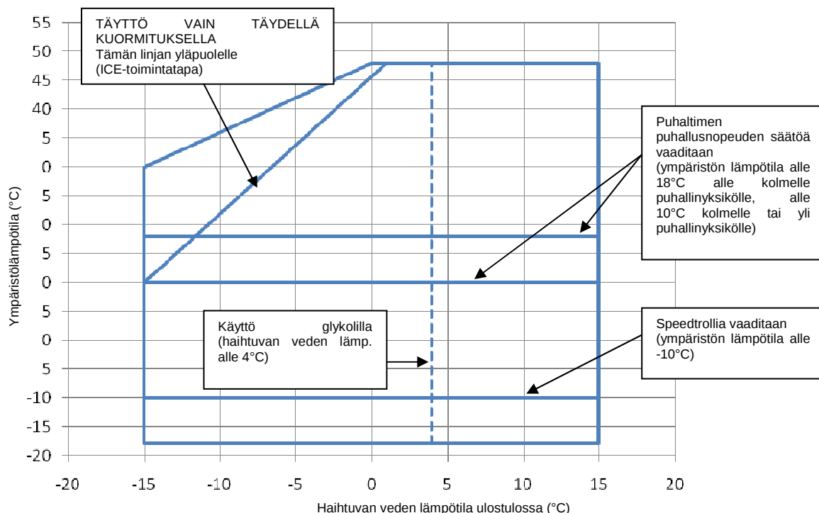
Kuva 2 – Käyttörajoitukset
