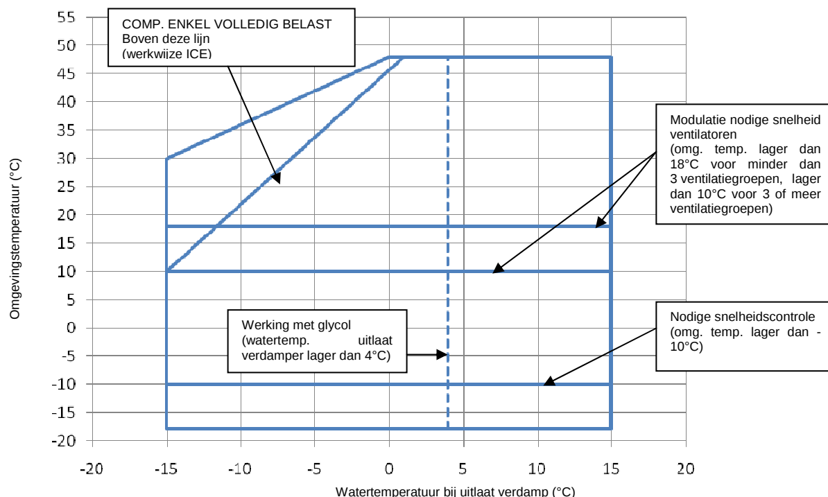
Figuur 2 – Werkingslimieten
