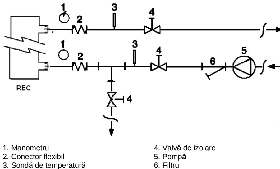
Figura 6 - Conectarea tuburilor de apă pentru schimbătoarele de recuperare a căldurii
