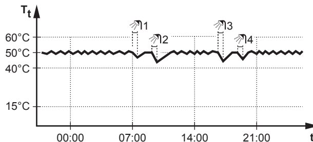
T t DHW katilo temperatūra t Laikas
